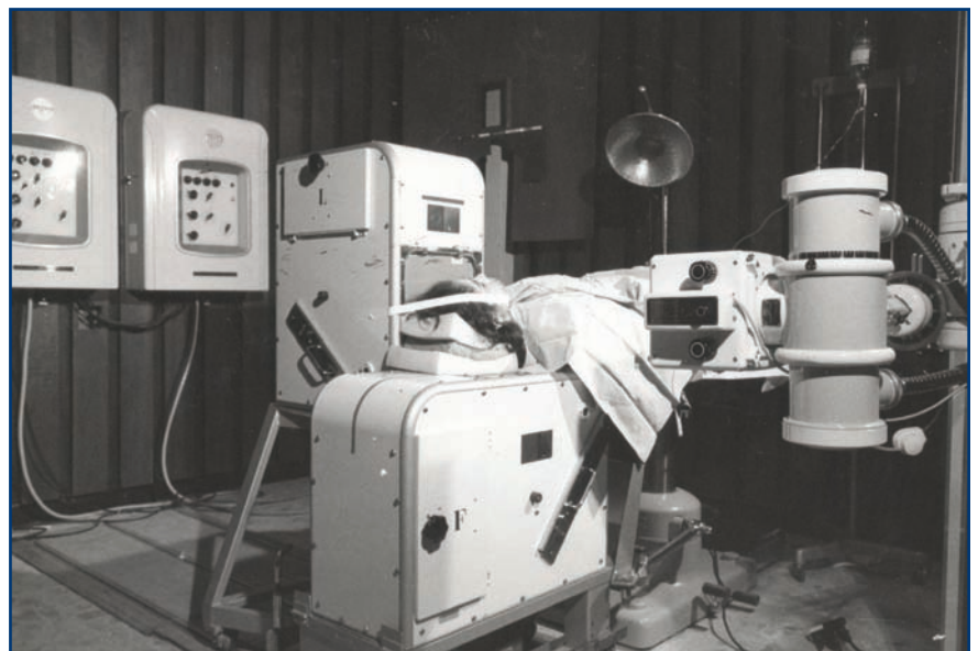
Imagen 11. Equipo AOT Elema Schnänder para realizar las angiografías cerebrales.
